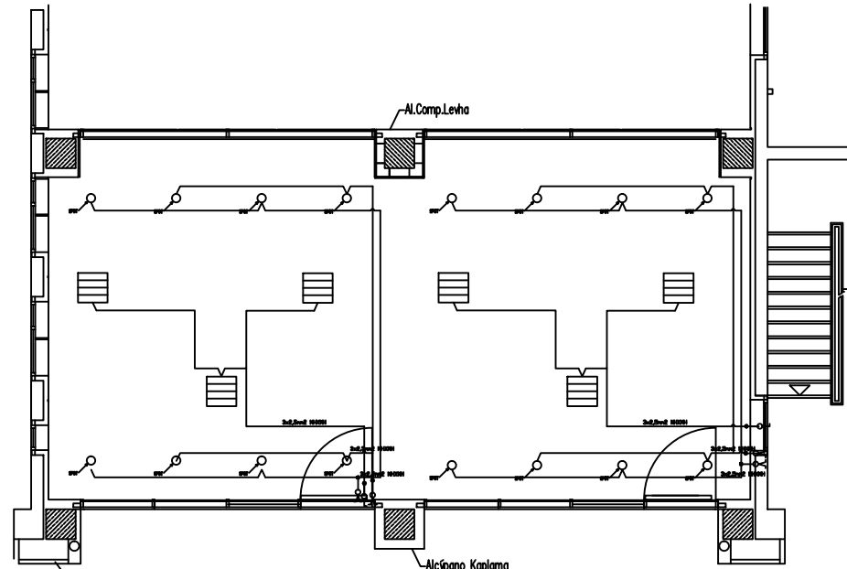
B-C BLOKLAR ARASI EK OFISLER 11-12-13 AKSLARI ZEMİN KAT
