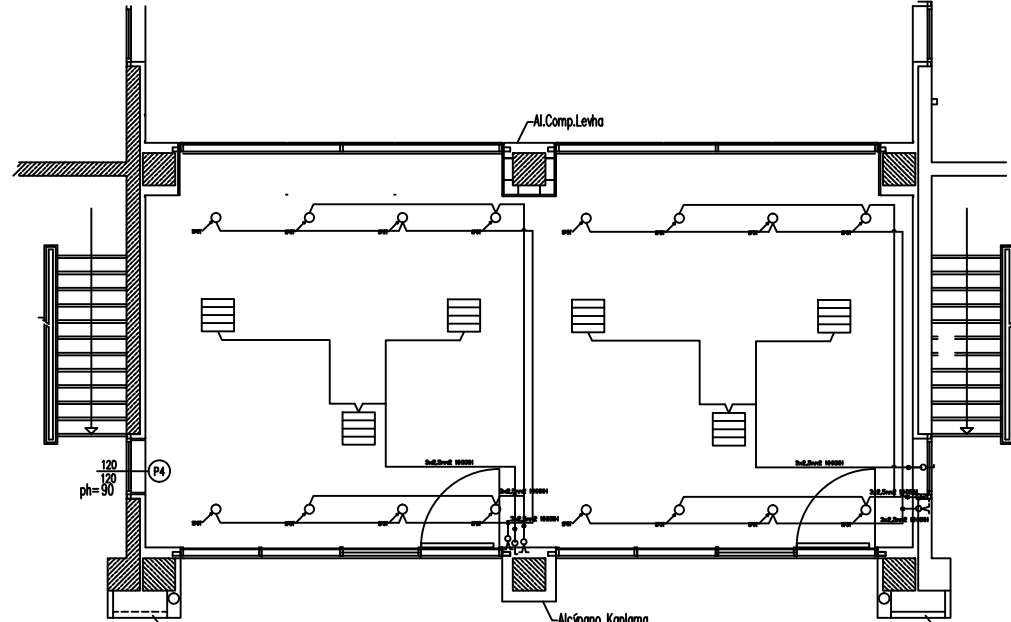
A-B BLOKLAR ARASI EK OFISLER 5-6-7 AKSLARI ZEMİN KAT
