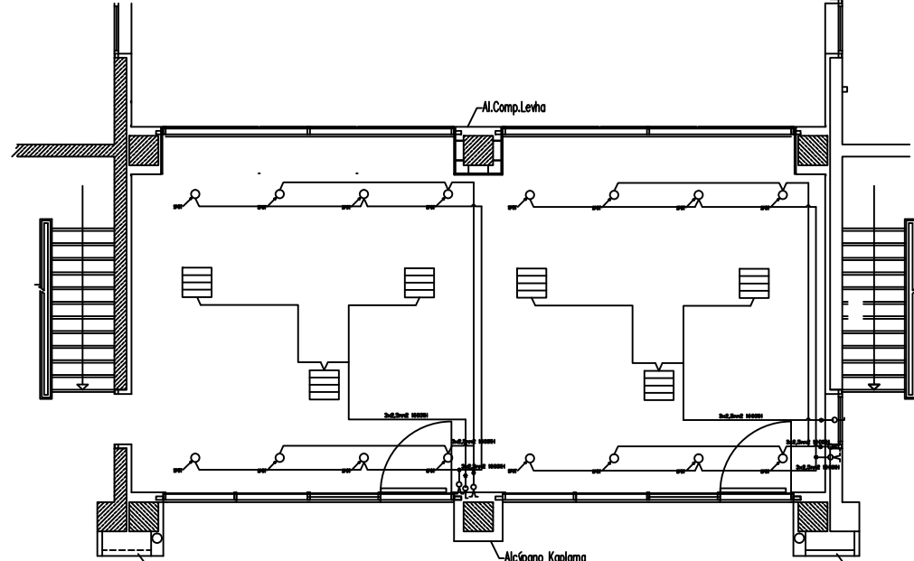
A-B BLOKLAR ARASI EK OFISLER 5-6-7 AKSLARI ASMA KAT
