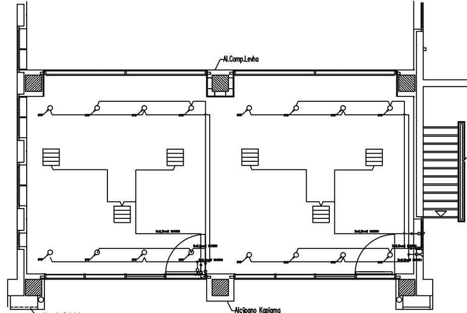
B-C BLOKLAR ARASI EK OFISLER 11-12-13 AKSLARI ASMA KAT
